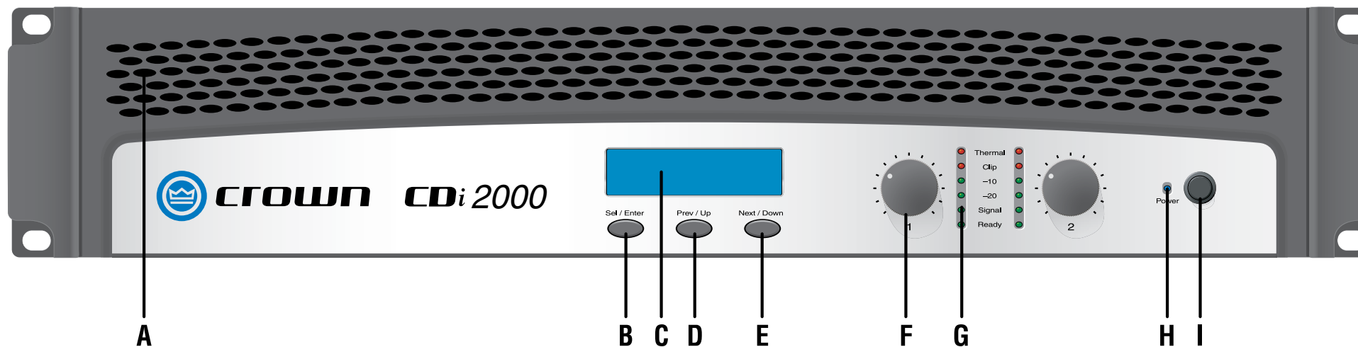
Figure 3.2 Commandes et indicateurs de façade
